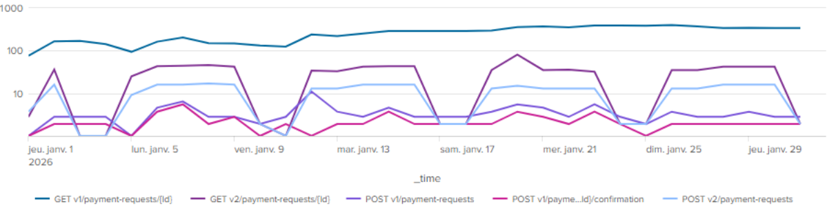
SANDBOX - Nombre appels par endpoint CBPII
