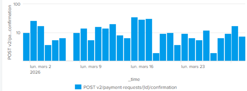
PISP - Nombre erreur 500 POST /payment-requests/{id}/confirmation
