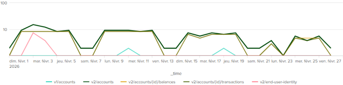
SANDBOX - Nombre appels par endpoint PISP
