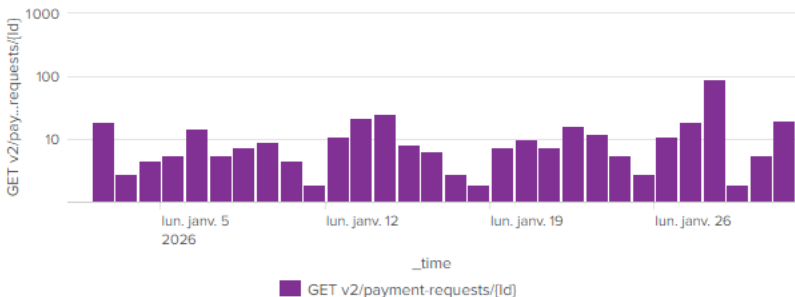
PISP - Nombre erreur 500 GET /payment-requests/{id}
