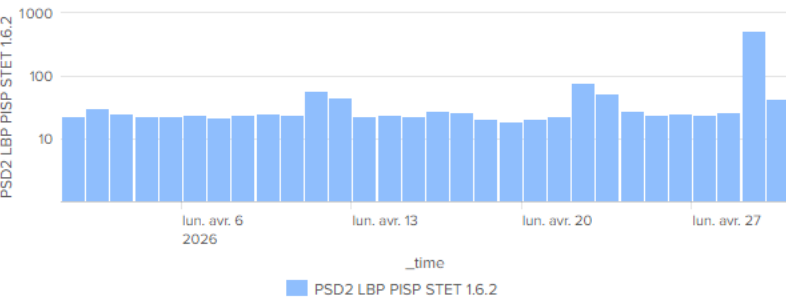
PISP - Nombre erreur 500 par API
