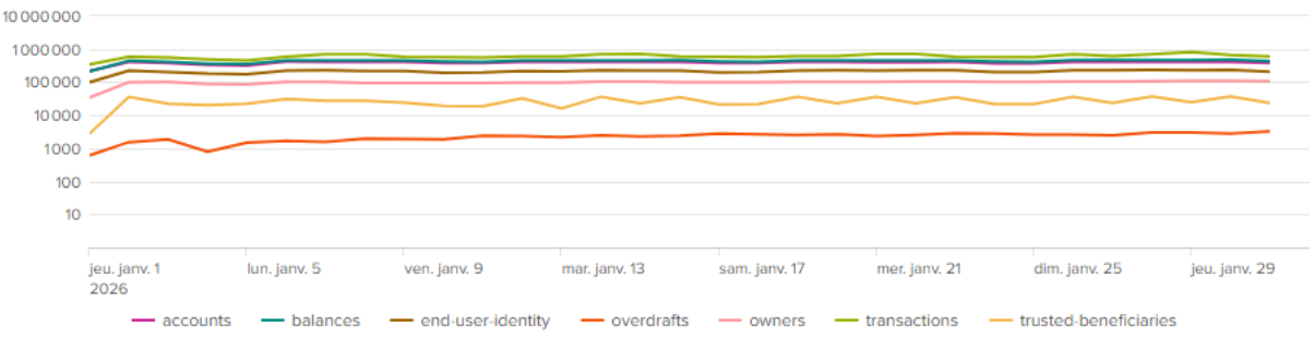
AISP - Nombre erreur 500 par endpoint
