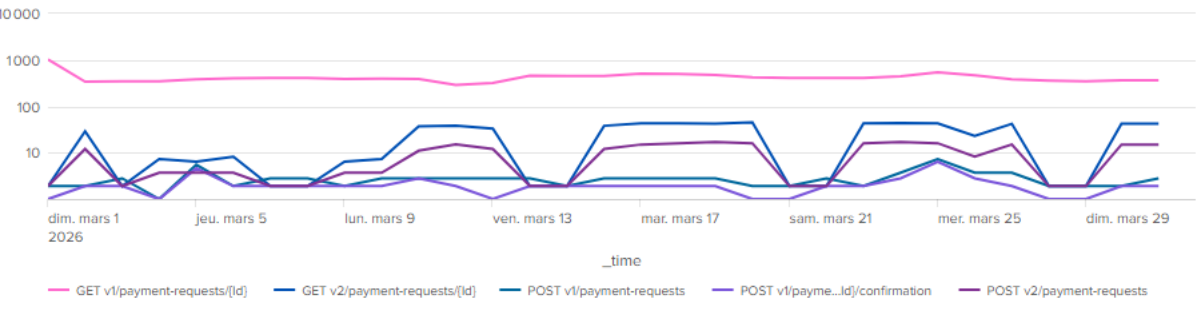
SANDBOX - Nombre appels par endpoint CBPII
