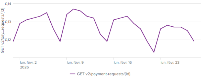
PISP - Temps de réponse GET /payment-requests/{id}
