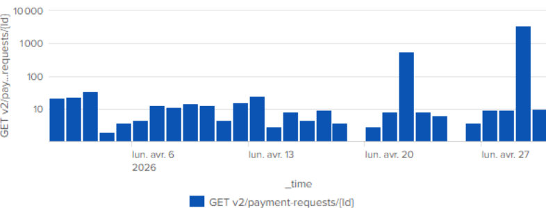
PISP - Nombre erreur 500 GET /payment-requests/{id}
