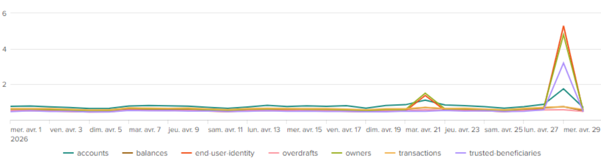
AISP - Temps de réponse par endpoint
