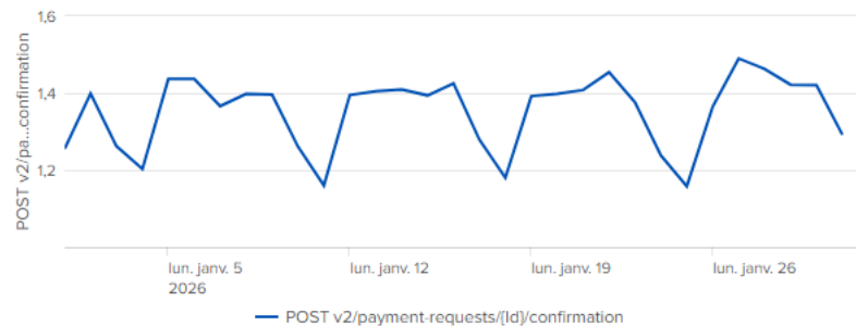
PISP - Temps de réponse POST /payment-requests/{id}/confirmation
