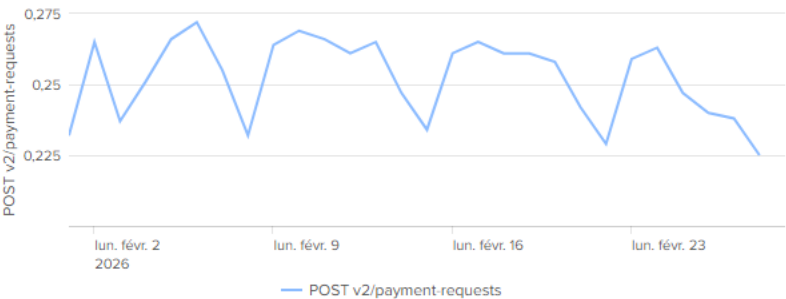
PISP - Temps de réponse POST /payment-requests
