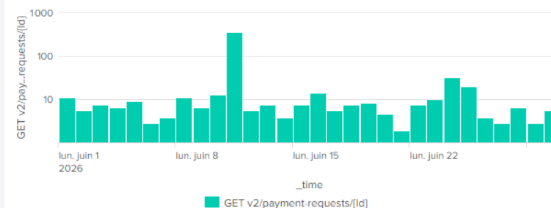
PISP - Nombre erreur 500 GET /payment-requests/{id}
