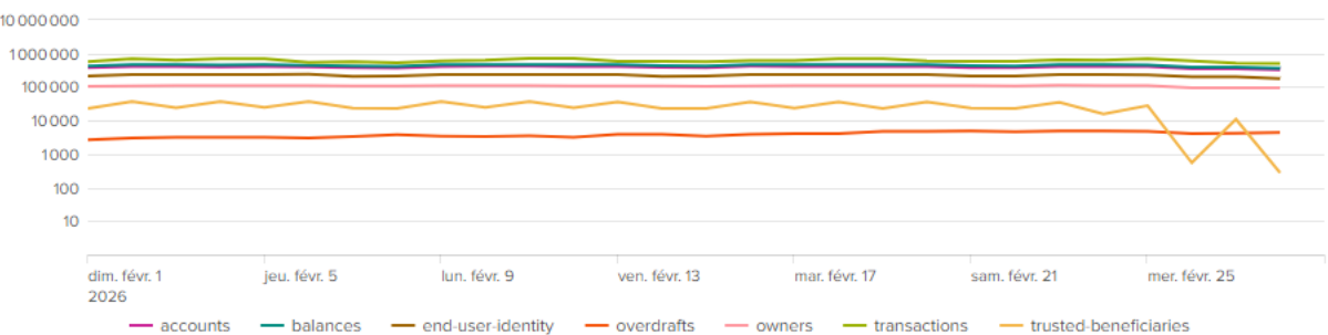
AISP - Nombre appels par endpoint
