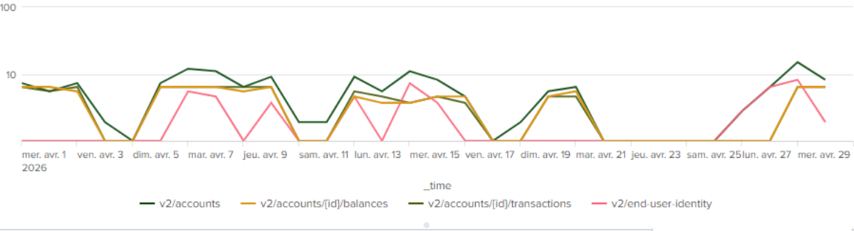
SANDBOX - Nombre appels par endpoint PISP
