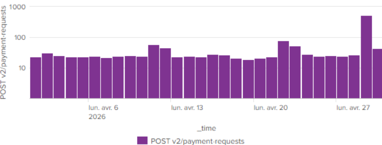
PISP - Nombre erreur 500 POST /payment-requests
